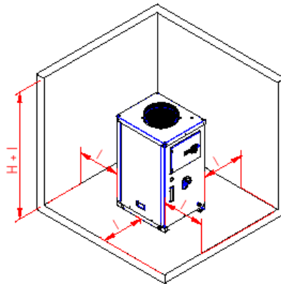
SPAZI DI RISPETTO I = 1000 mm
